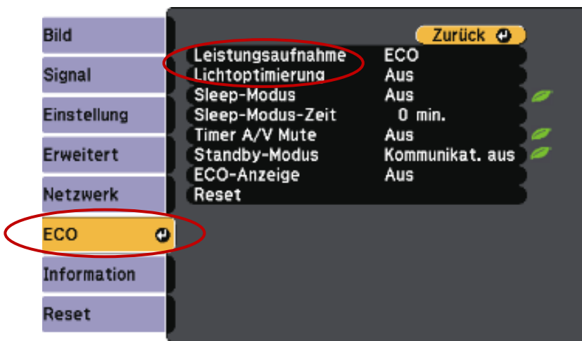
Beispiel: Beamer-Menu
